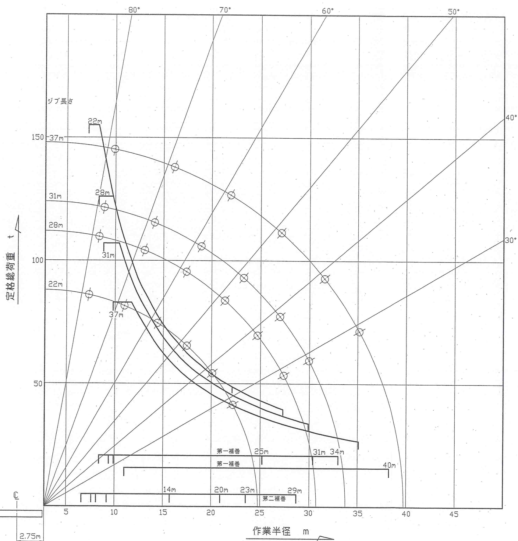
155tフック、50tフック、20.7tフック、5tフック 使用時 総合
